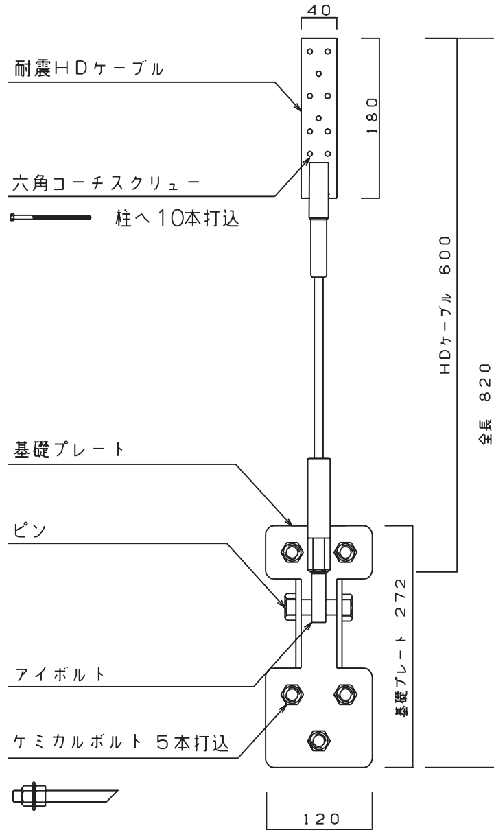
正面図
