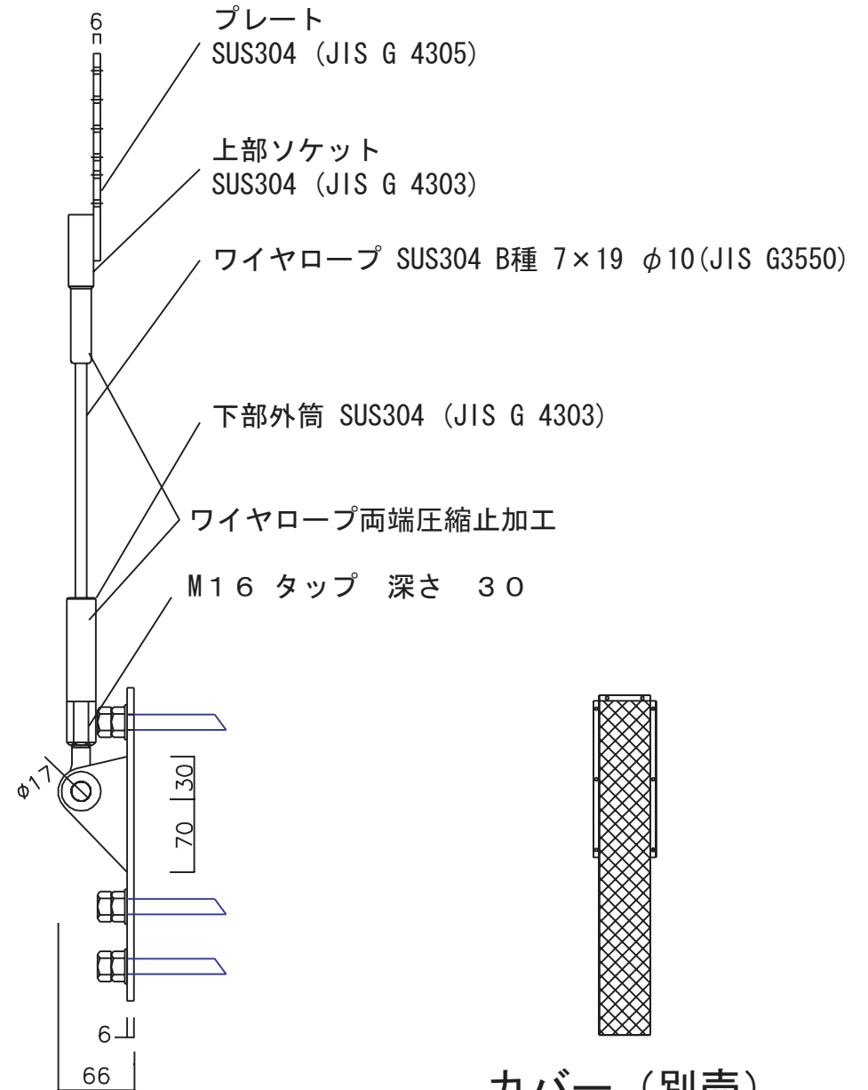
側面図
